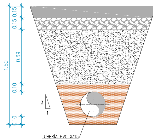
TUBERÍA PVC Ø315
