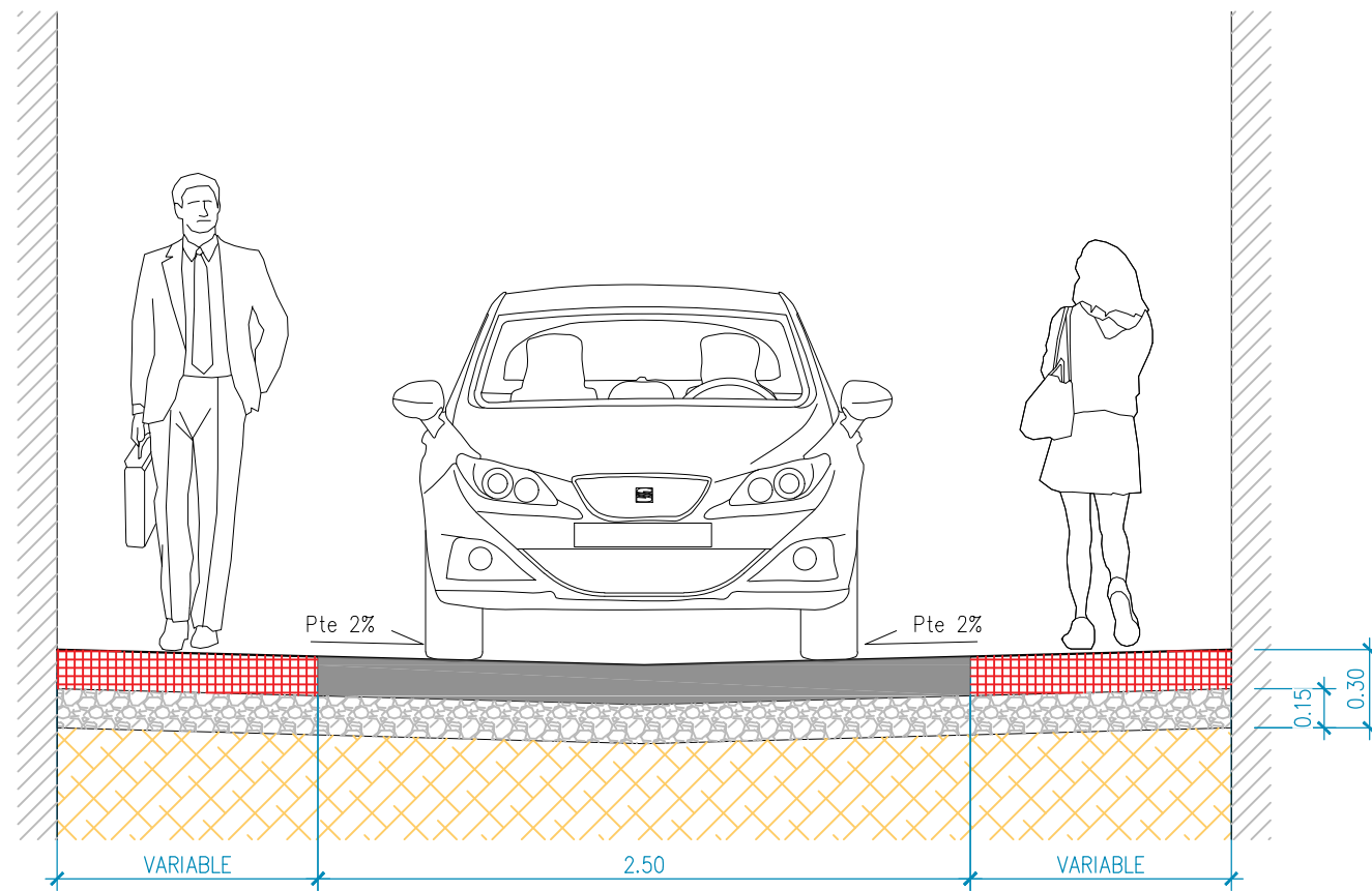
SECCIÓN TIPO
