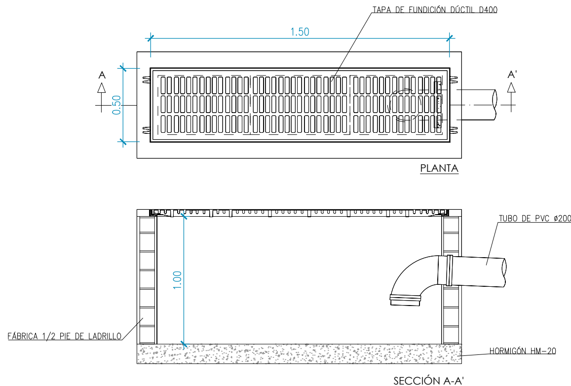
SECCIÓN A-A'
