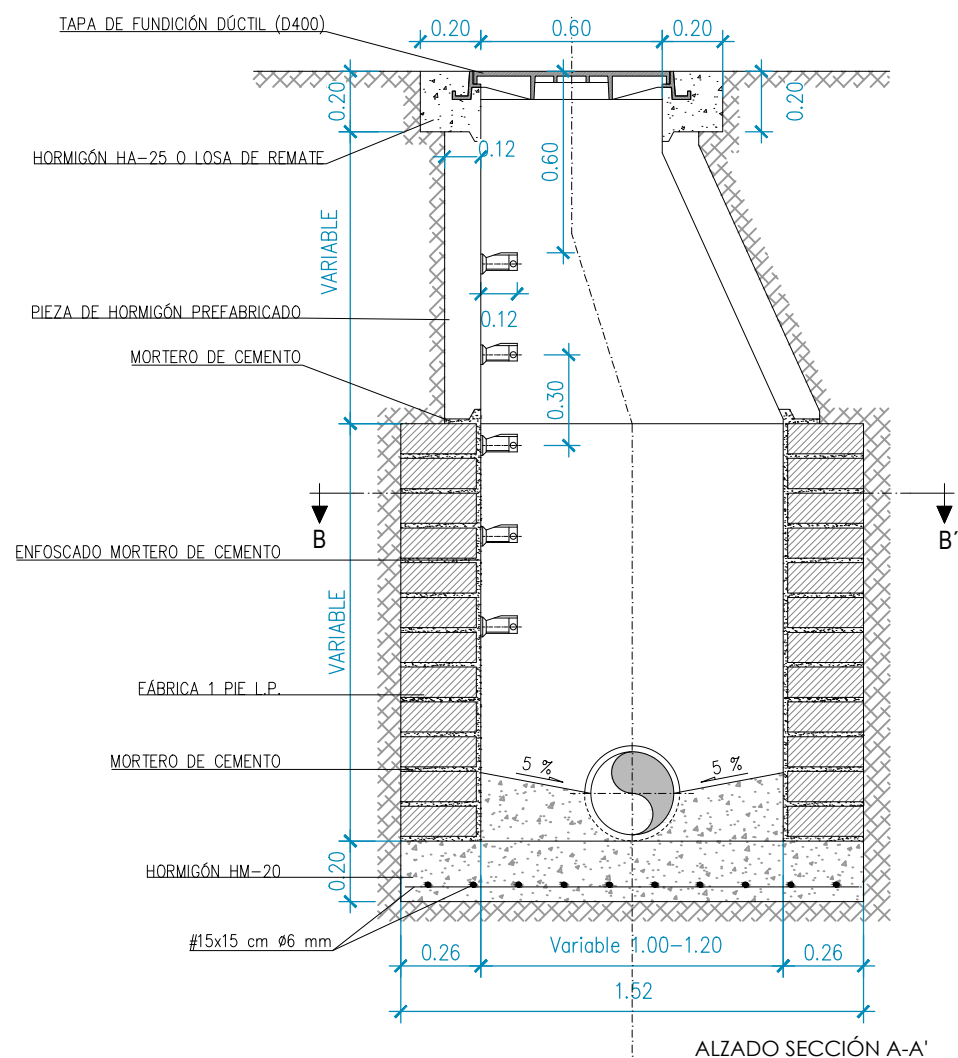
ALZADO SECCIÓN A-A'
