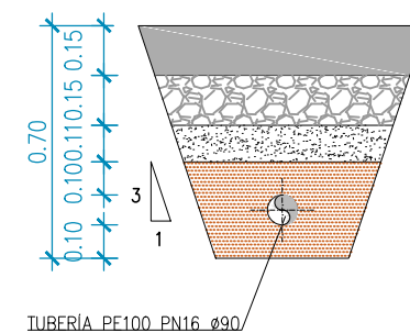
TUBERÍA PE100 PN16 Ø90
