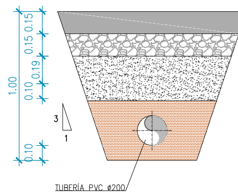
TUBERÍA PVC Ø200
